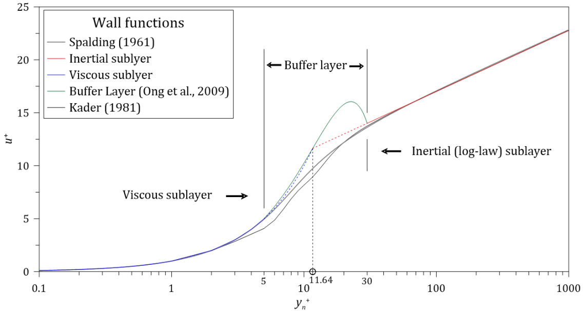
그림 A.1. Wall functions in turbulent boundary layer
