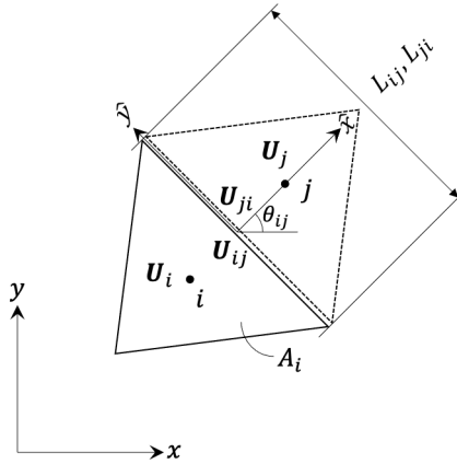
그림 1. Local Coordinate System (\hat{x}, \hat{y})
